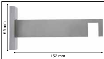
Soporte Largo
