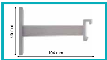
Soporte Frontal
