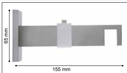
Soporte Doble
