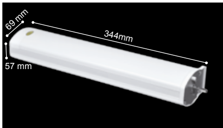
Motor RM09-92
